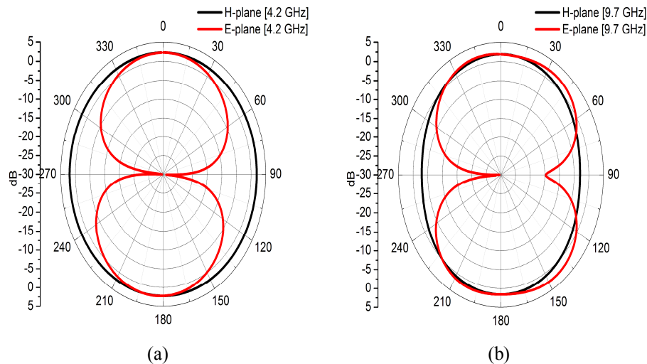
Fig. III.10. Diagrammes de rayonnement simulés et mesurés à : (a) 4.8 GHz et (b) 9.7 dans le plan XZ et plan YZ.
