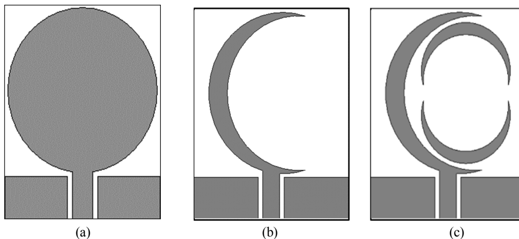
Fig. IV.10. Évolution de l'antenne fractale proposée. (a) La géométrie de base circulaire, (b) Première itération et (c) Deuxième itération.
