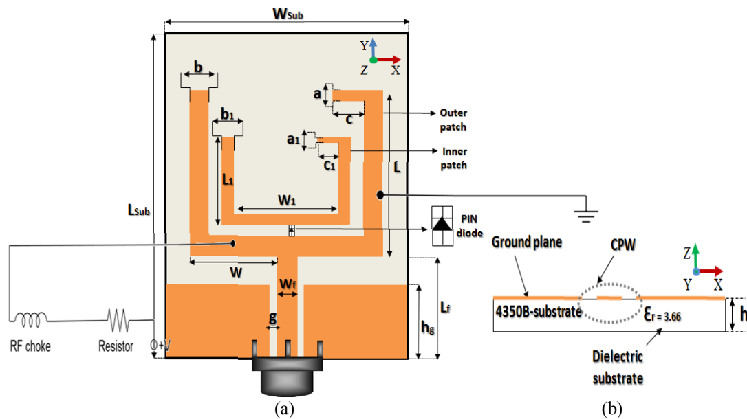
Fig. V.3. Schéma de l'antenne proposée avec le switch réel : (a) vue de dessus, (b) vue de dessous.
