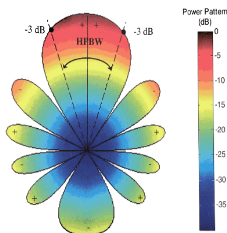
Fig. I.6 Exemple de diagramme de rayonnement normalisé à deux dimensions en dB [I.3].
