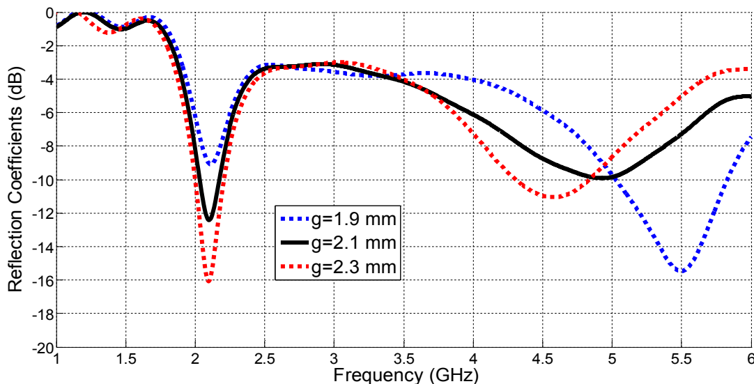
Fig. IV.14. Variation du coefficient de réflexion en fonction de la fréquence tenant compte de l'effet du gap 'g' de la ligne CPW.
