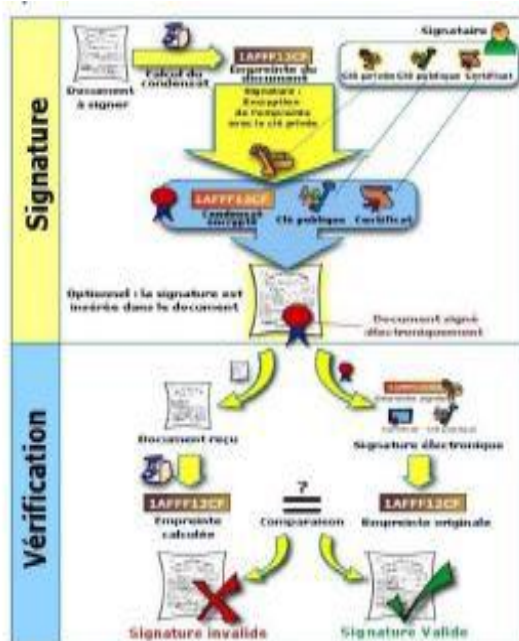
- شكل يوضح آلية التحقق من التوقيع - 2
