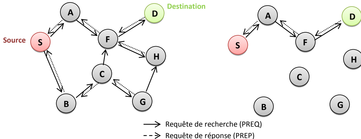
Figure 2.5 Propagation de la requête de recherche d'une route
