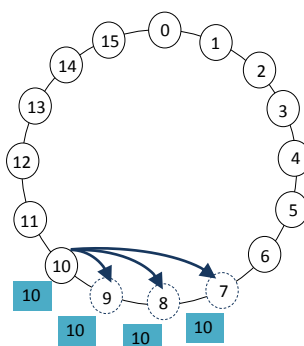
Figure3.1 La réplication proposée, appliquée sur la clé 10 ( m=4, r=3 )
